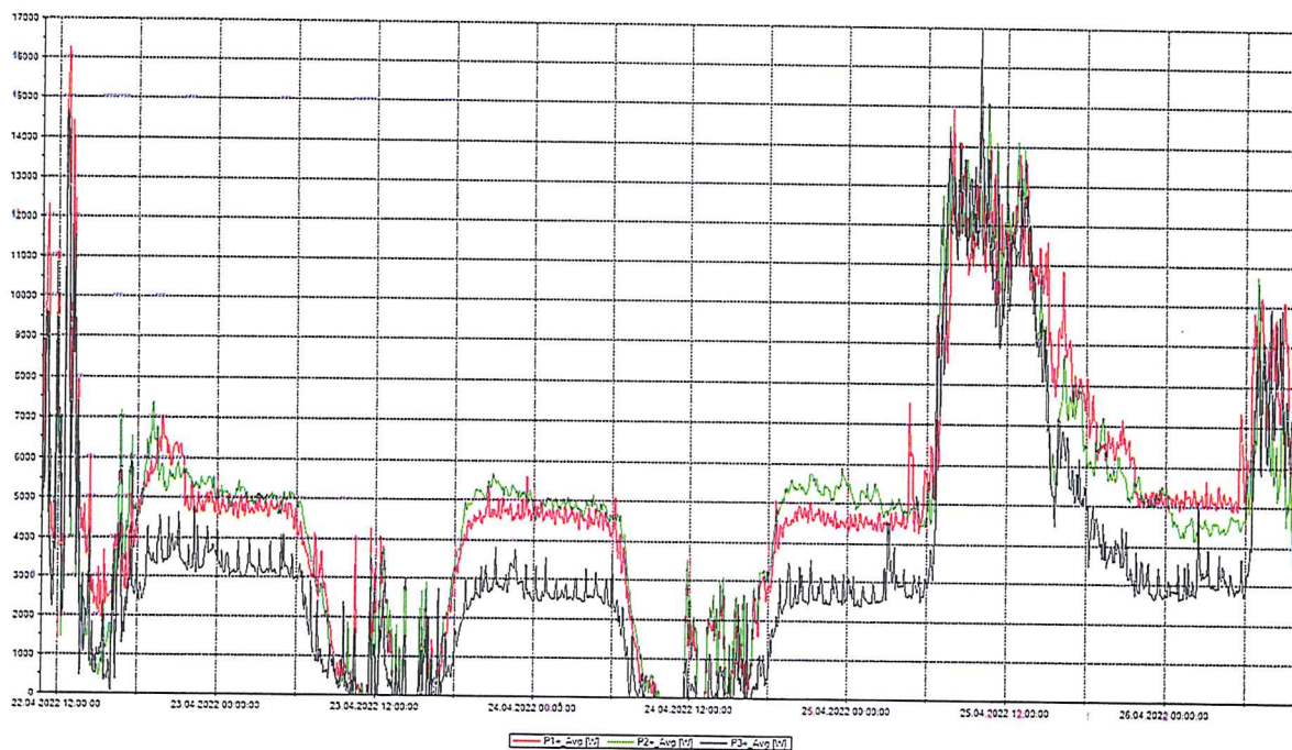
Wykres 6. Moc czynna w fazach
